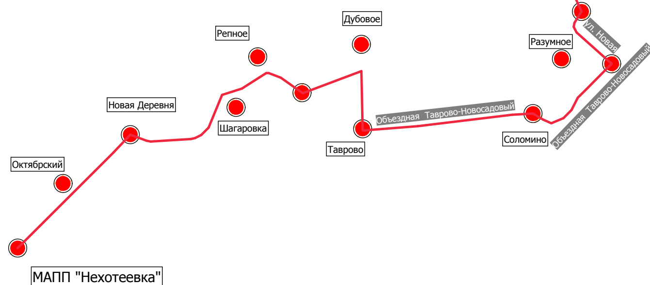
Транспортно-логистическая схема движения транспортных средств от пограничного пункта пропуска: МАПП "Нехотеевка"
