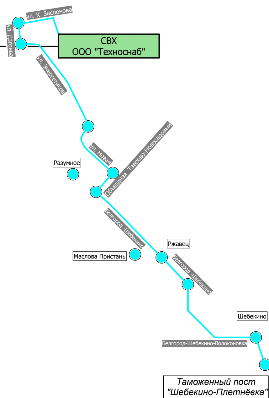
Транспортно-логистическая схема движения транспортных средств от пограничного пункта пропуска "Шебекинский" им. В.А. Данкова
